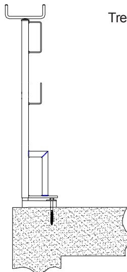
Befestigung mit Dübel und Schraube
