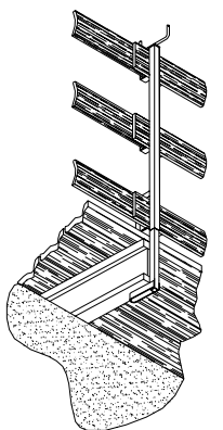
Ausschussgerüste
